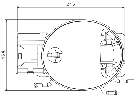
俯视图
