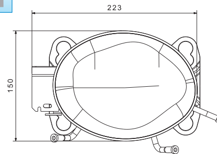
俯视图
