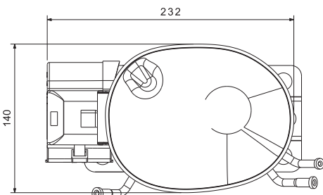
俯视图
