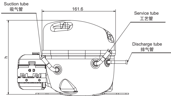
主视图
