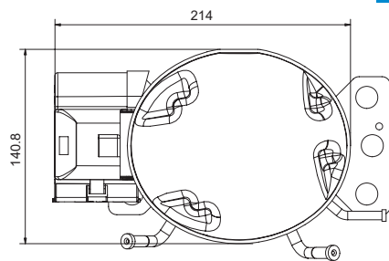
俯视图
