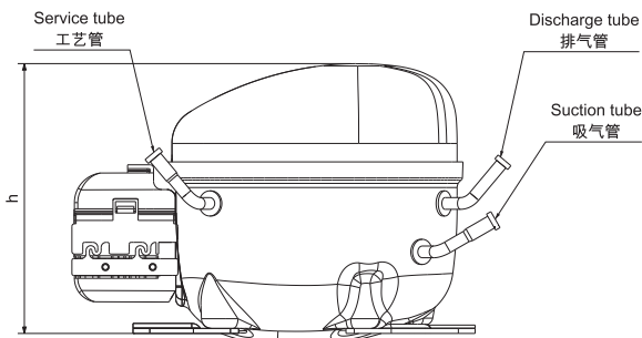
主视图
