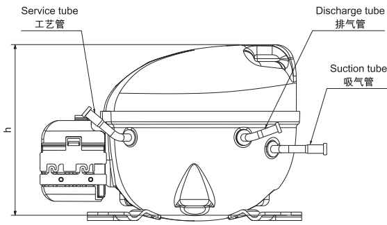
主视图
