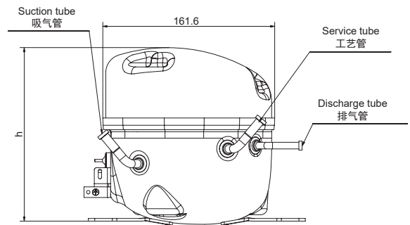
主视图
